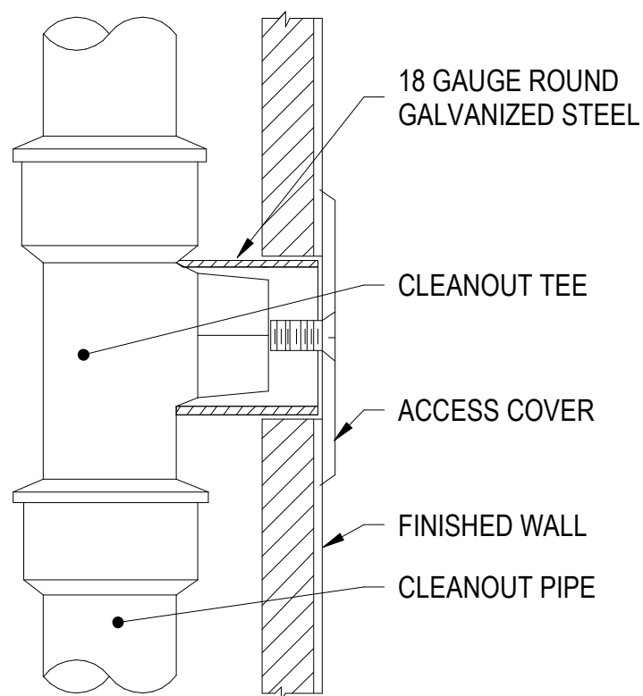
5 WALL CLEANOUT SCALE:NTS
